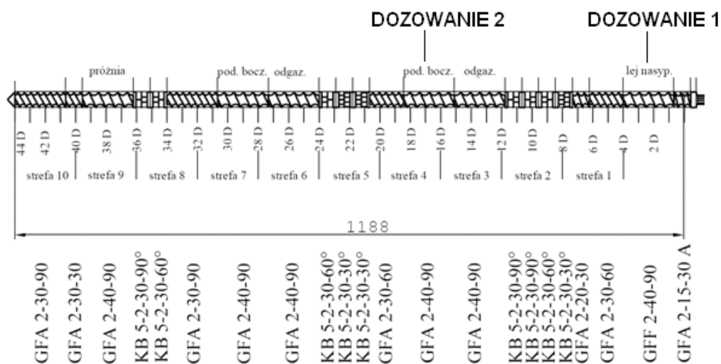
Rys. 1. Konfiguracja ślimaków
