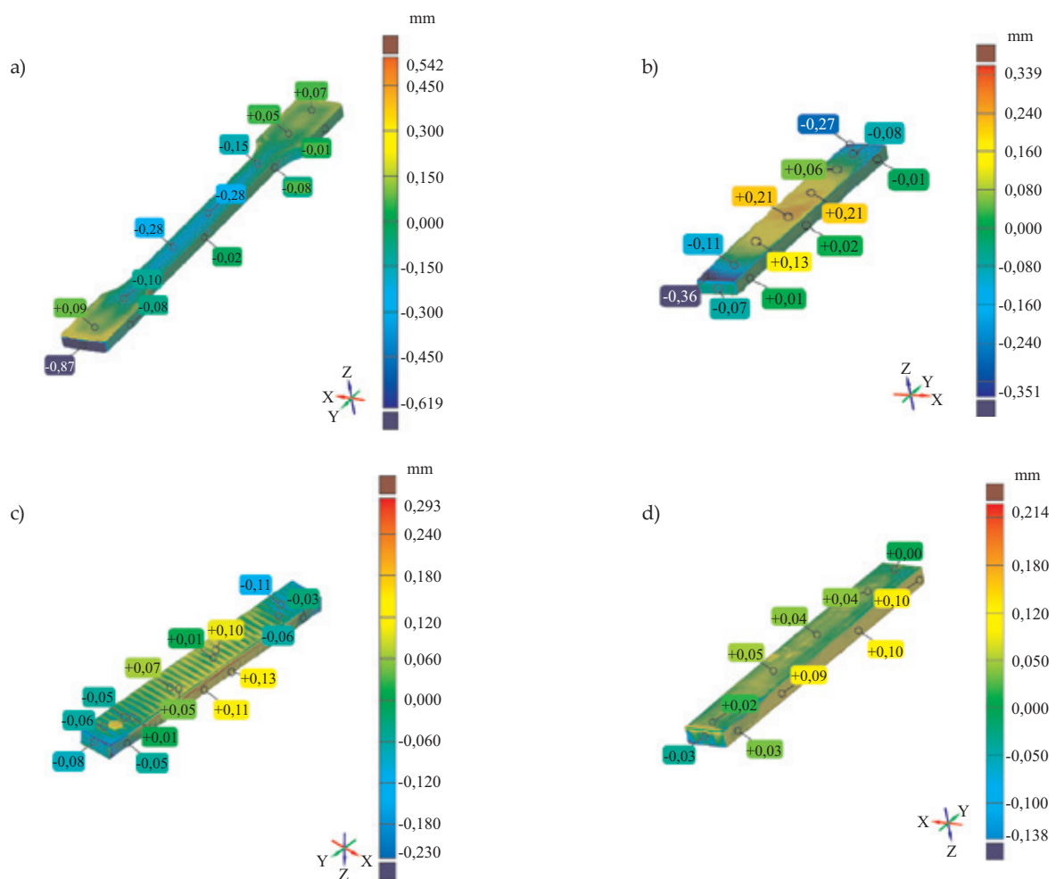
Rys. 8. Porównanie mapy odchyłków wymiarowych próbki wtryskiwanej (a) oraz wybranych próbek różniących się grubością warstwy i kątem orientacji: 0,254 mm, 0° (b); 0,254 mm, 45° (c) oraz 0,178 mm, 90° (d)
